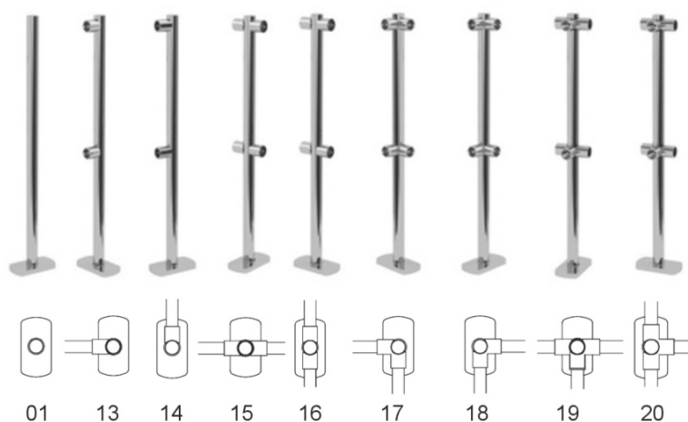
Configurations complètes de poteaux H-1085 mm (poteaux avec cache inférieur et jonctions):
