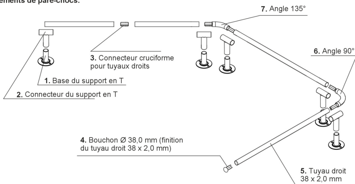
Schéma des éléments de pare-chocs:
